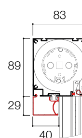
CASSONETTO 80 MM
