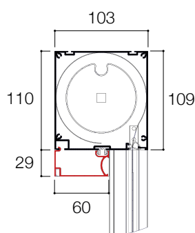
CASSONETTO 100 MM
