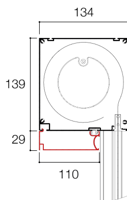
CASSONETTO 130 MM
